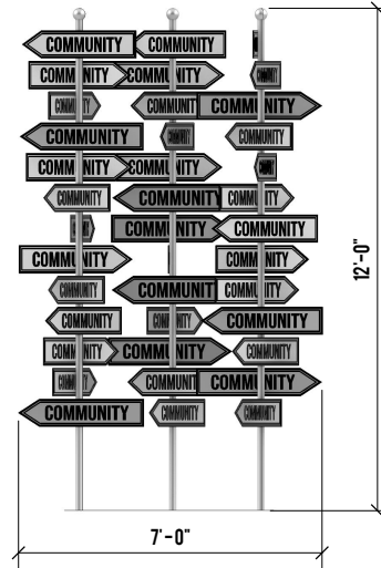
ELEVATION
